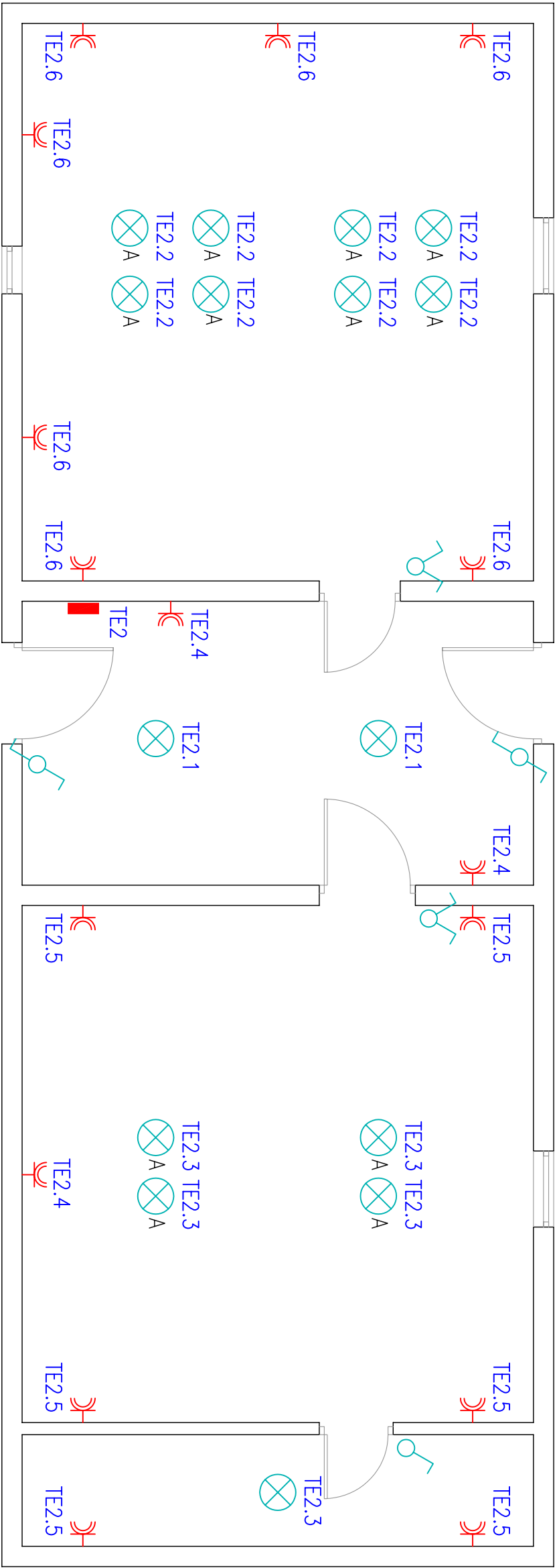
RZUT PRZYZIEMIA
